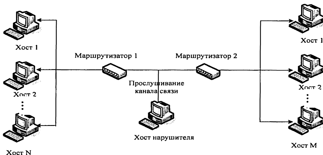
Рисунок 6. Схема реализации угрозы "Анализ сетевого трафика"
