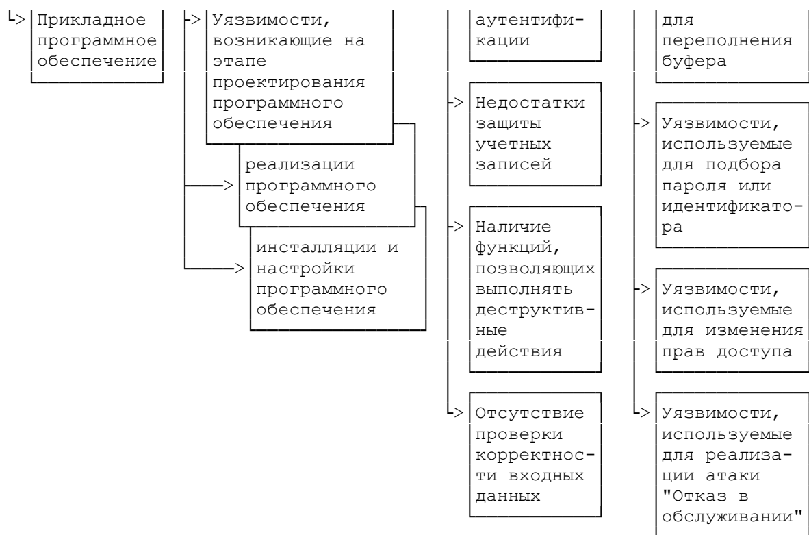
Рисунок 4. Классификация уязвимостей программного обеспечения
